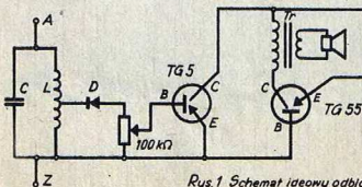
Rys.1 Schemat ideowy odbiornika
